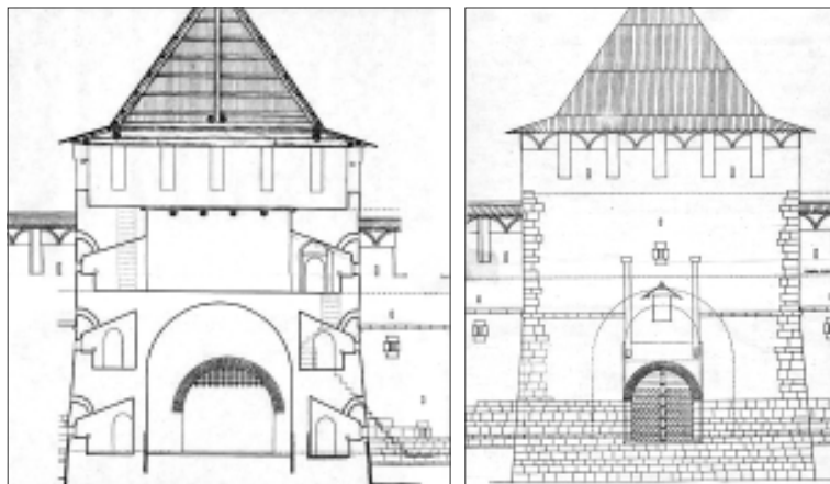
Реконструкция первоначального облика Зачатьевской башни. Разрез и северный фасад. (Арх. И.С. Агафонов)
